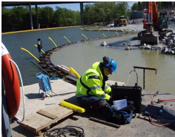
Installation av inklinometrar på spont
